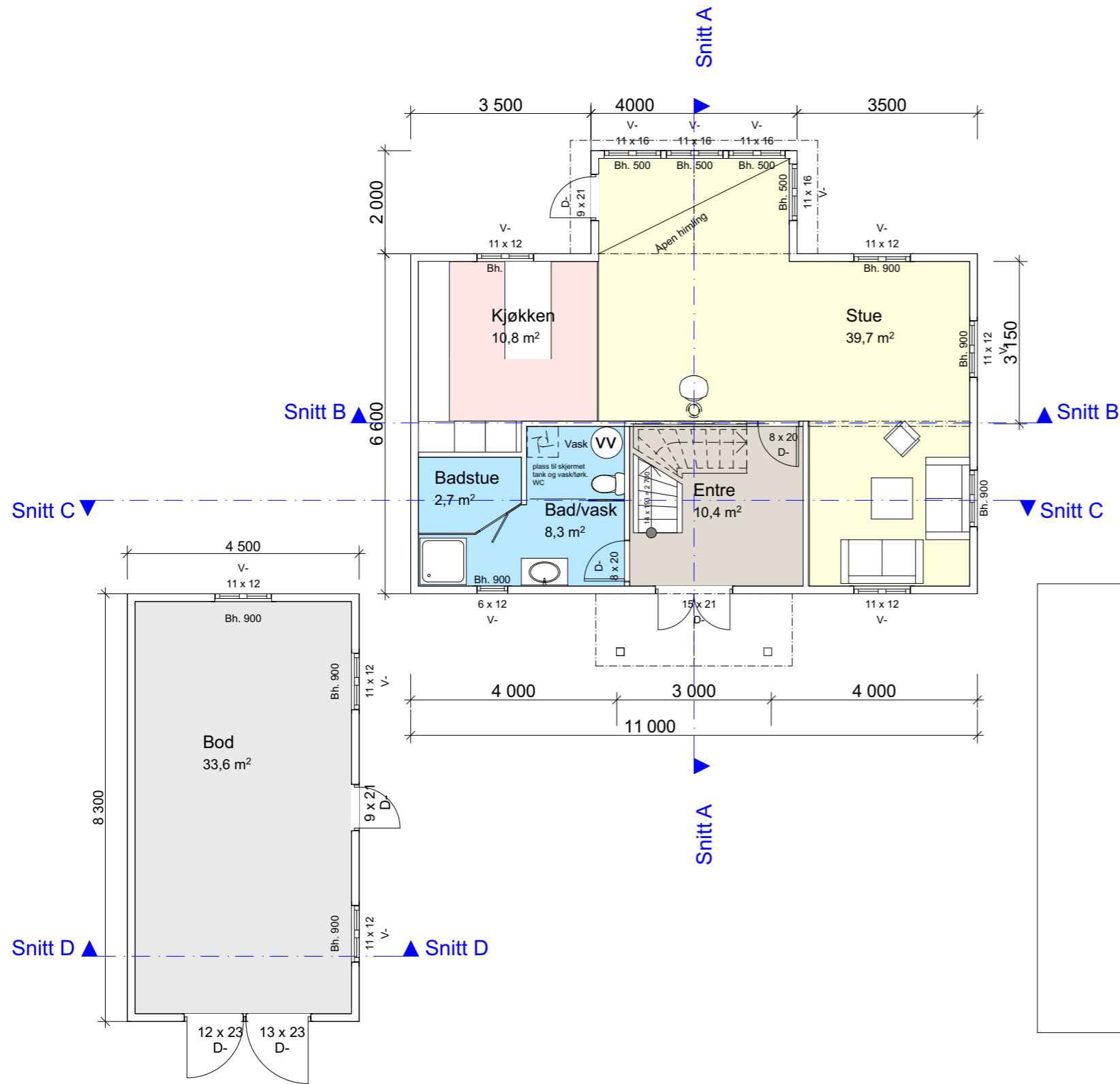
1.PLAN.
