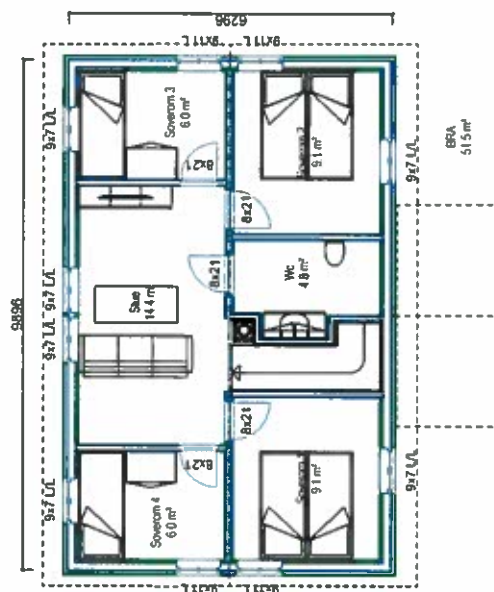
Plan 2.Etg.
