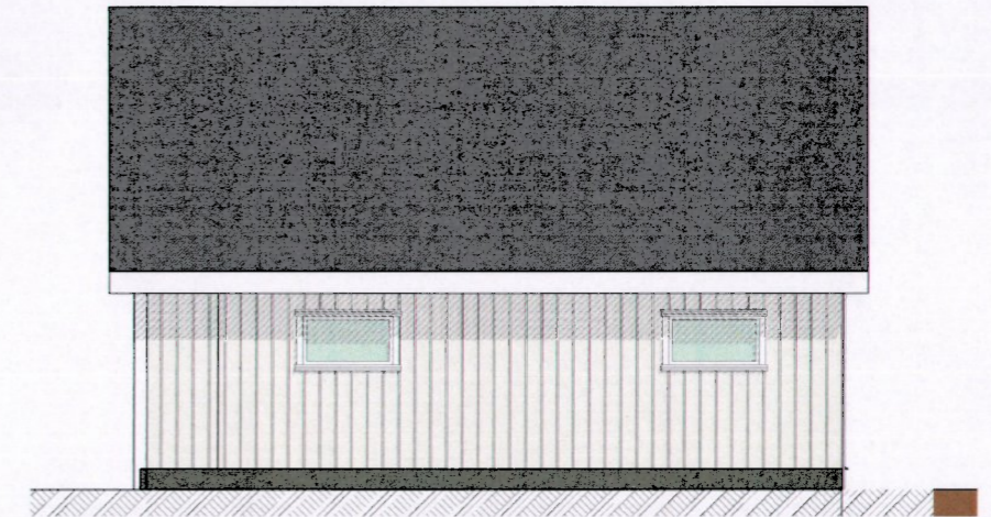
Fasade 4
