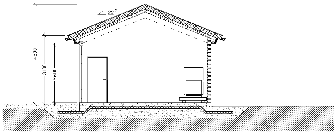
SNITT A-A
