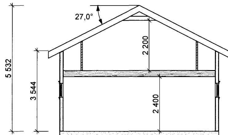
SNITT A-A
