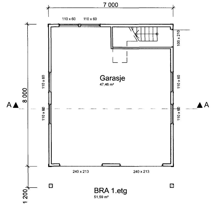
PLAN 1.ETG.
