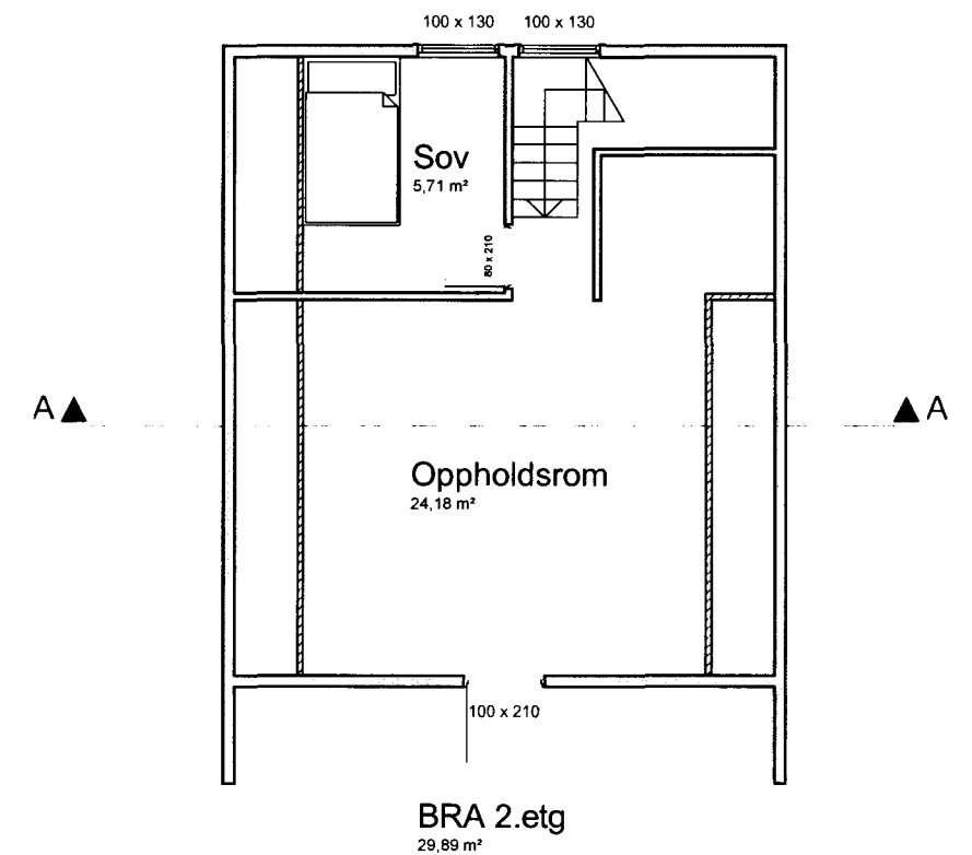
PLAN 2.ETG.
