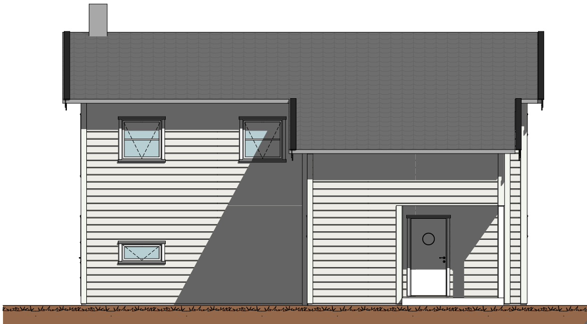
Fasade 3
