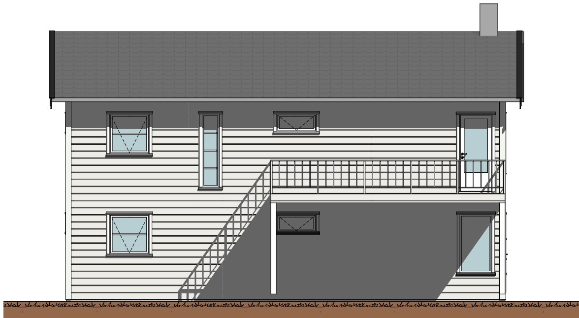
Fasade 1
