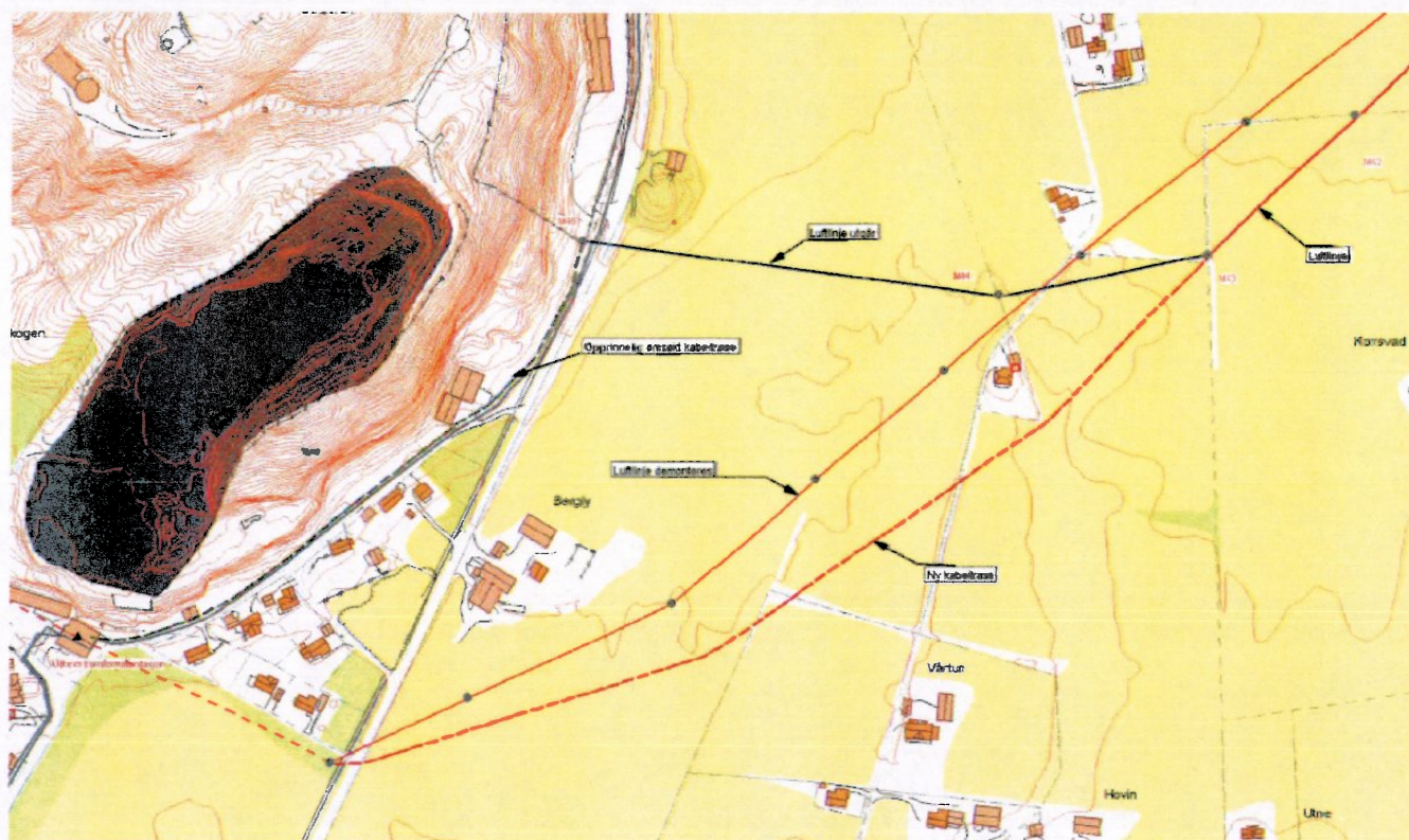
Figur 1 - Kart som viser omsøkte endring. Sort stiplet og hel strek viser tidligere konsesjonsgitte kabel- og luftledningstrasé. Rød stiplet linje viser ny kabeltrasé.
