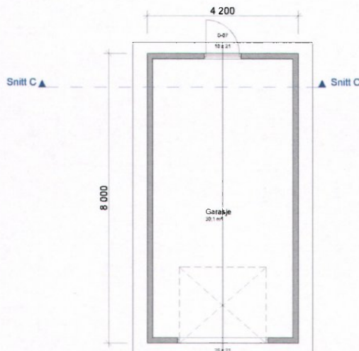
Plan 1:100
