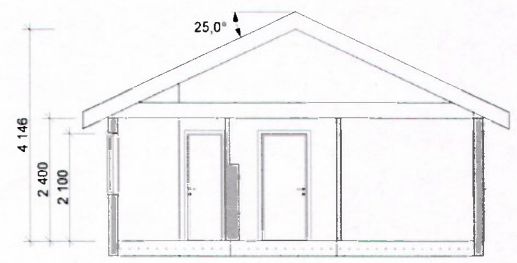
Snitt A
