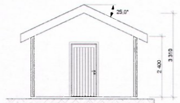
Snitt C 1:100
