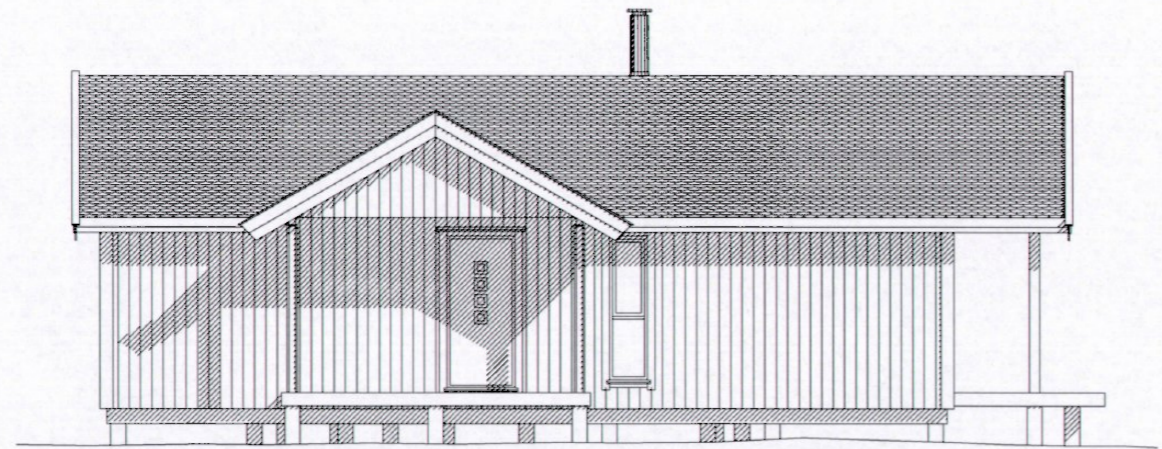
Fasade 3
