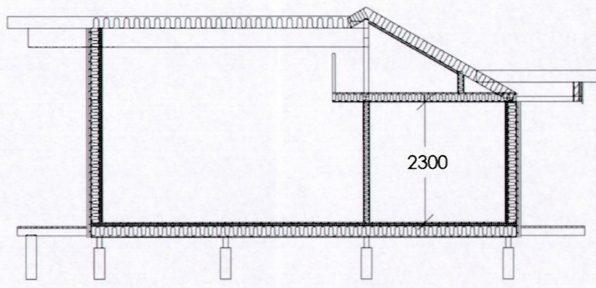
Snitt B-B
