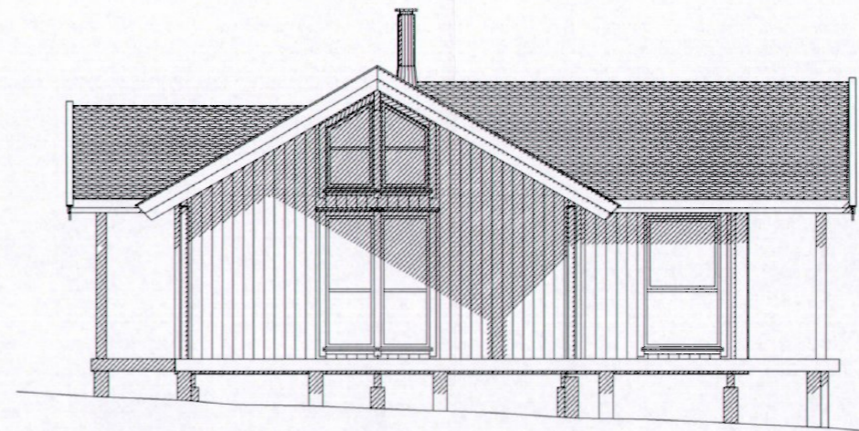
Fasade 4
