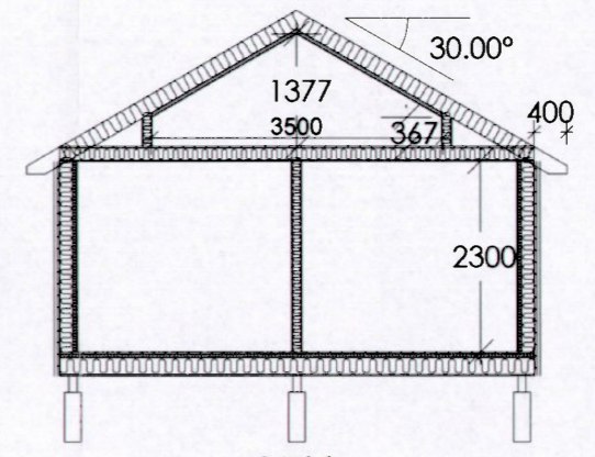
Snitt C-C
