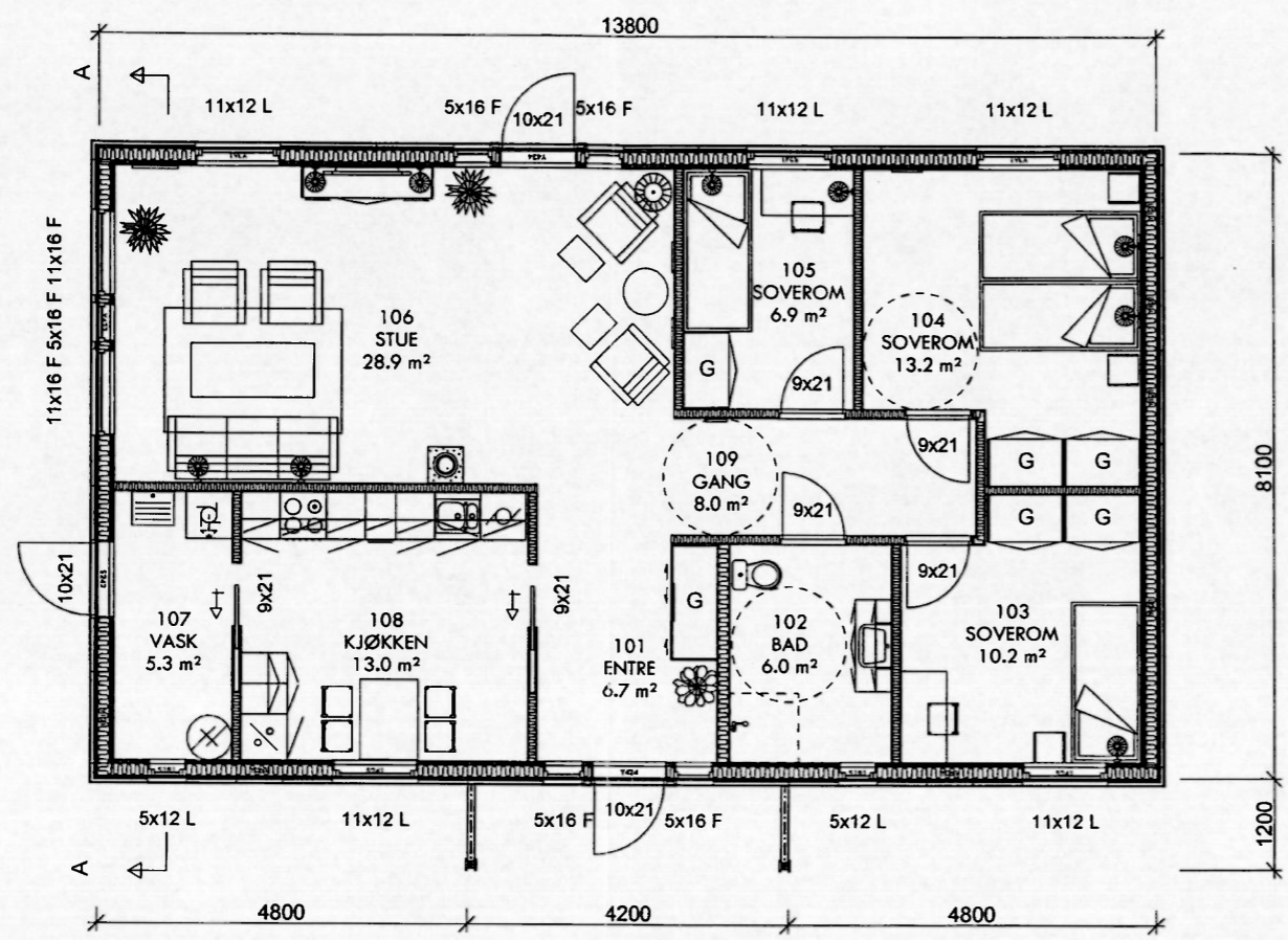
HOVEDPLAN
