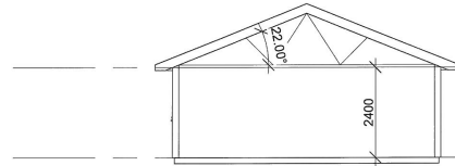
Section 1 1 : 100
