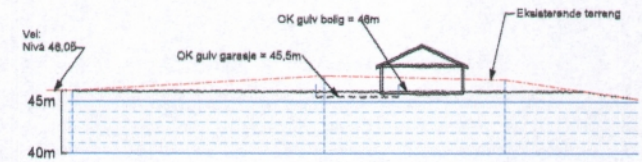
Snitt 26
