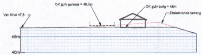
Snitt 25
