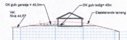
Snitt 27
