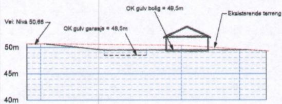
Snitt 24
