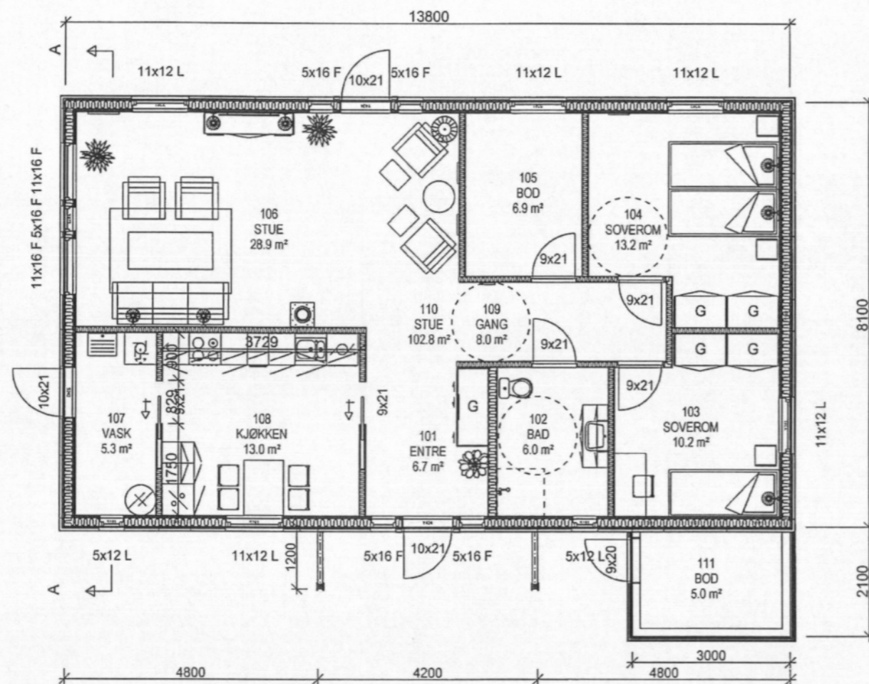
HOVEDPLAN
