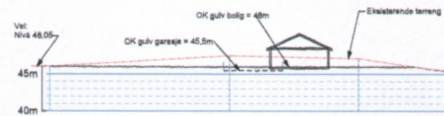
Snitt 26
