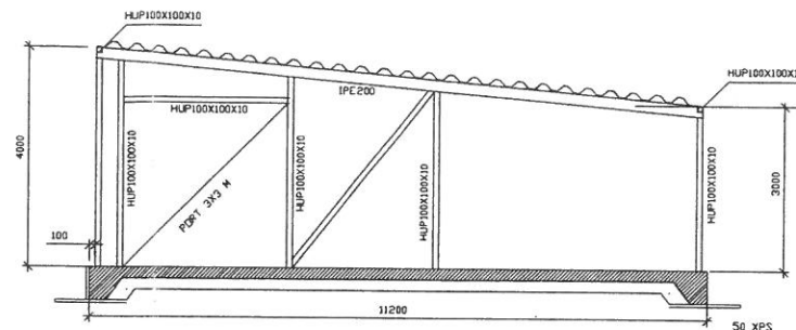
OPPRISS FASADE AKSE 3
