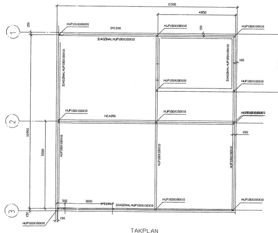
TAKPLAN
