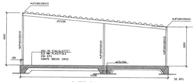
SNITT B
