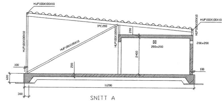
SNITT A
