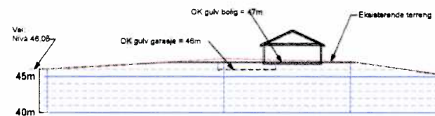
Snitt 26
