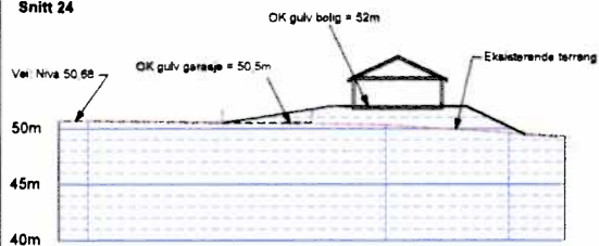
Snitt 24
