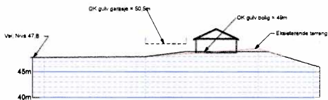
Snitt 25
