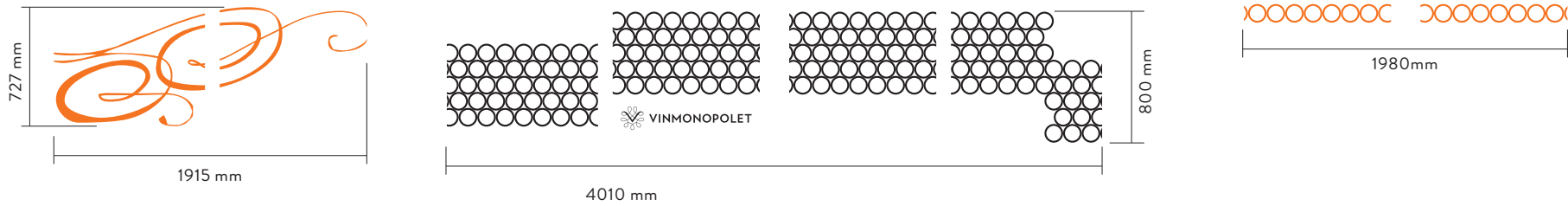
Skala 1:40 (A4)
