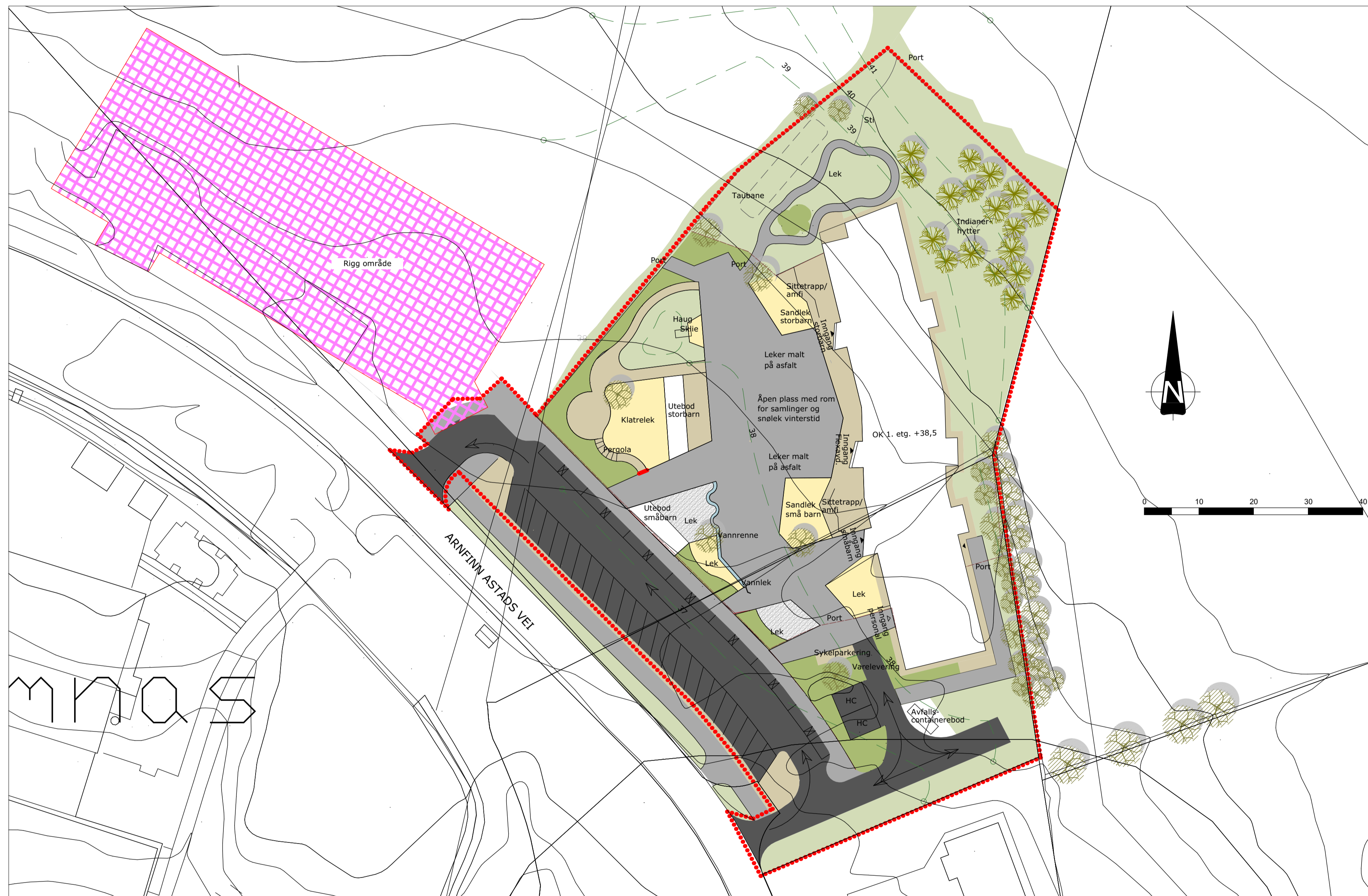
Utomhusplan 1:500
